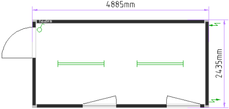
16-и футовый офисный блок-контейнер
